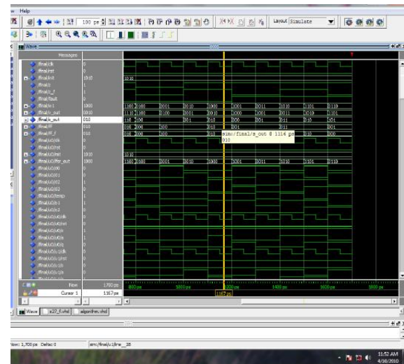
Fig.7. Fault free Final Module
